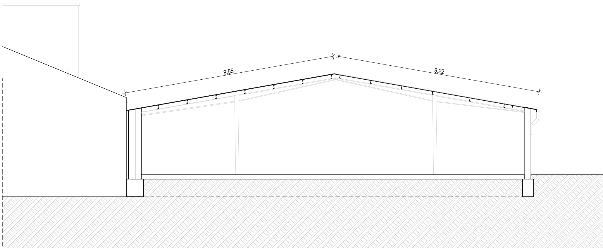
A-A METSZET, M=1:100
